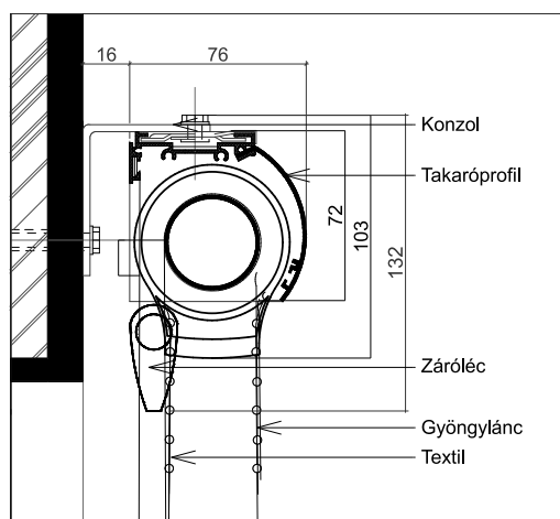
Oldalfali szerelés
