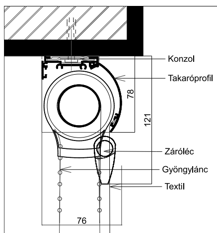
Mennyezeti szerelés
